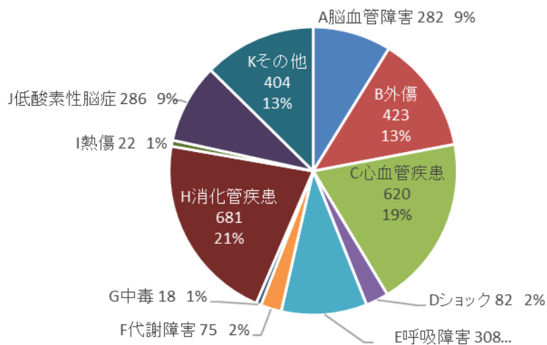
疾患別分類
